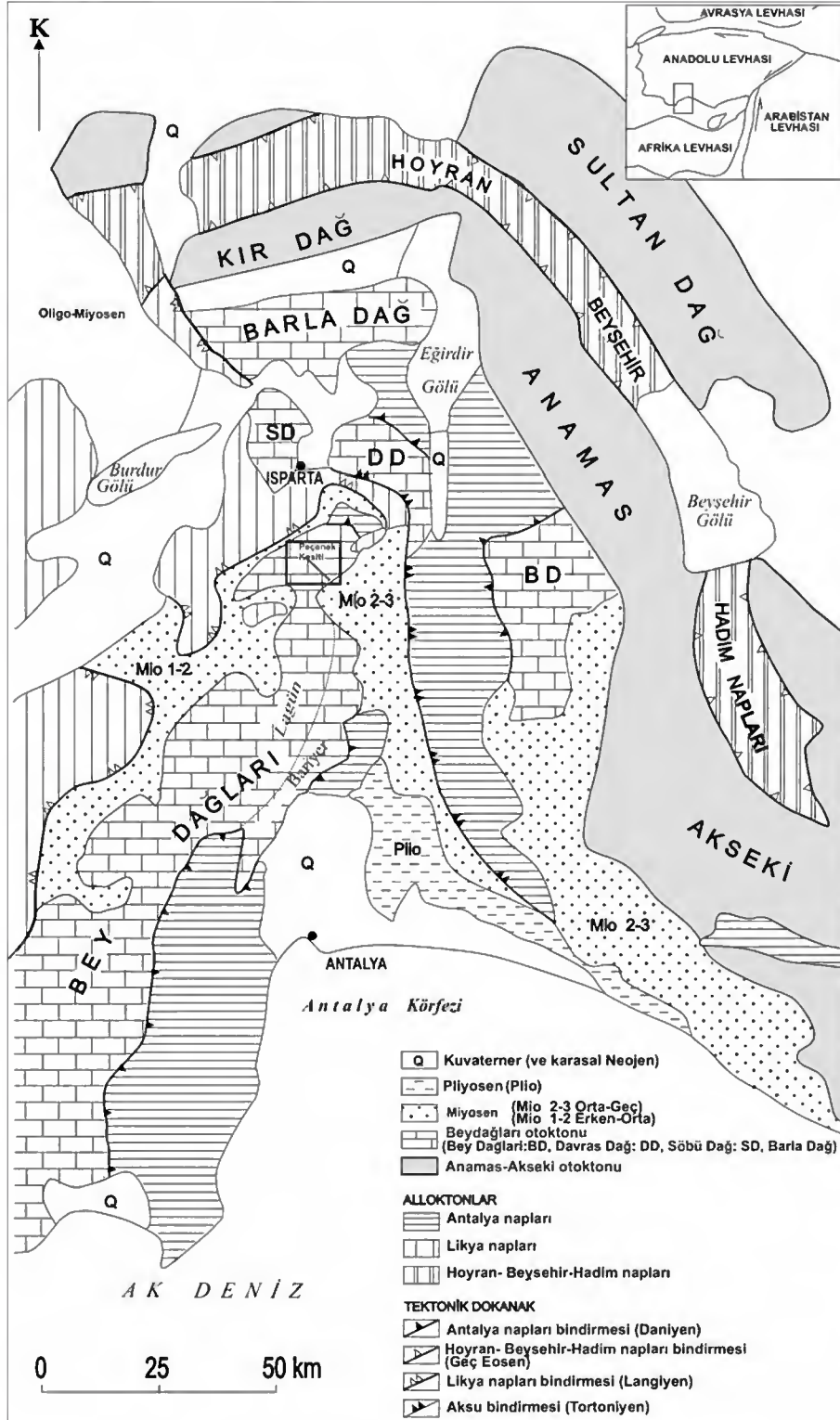
Şekil 1. Çalışma alanının jeolojik konumunu gösterir harita (PK: Peçenek Boğazi Kesiti) (Poisson et al., 2003' den düzenlenmiştir).
