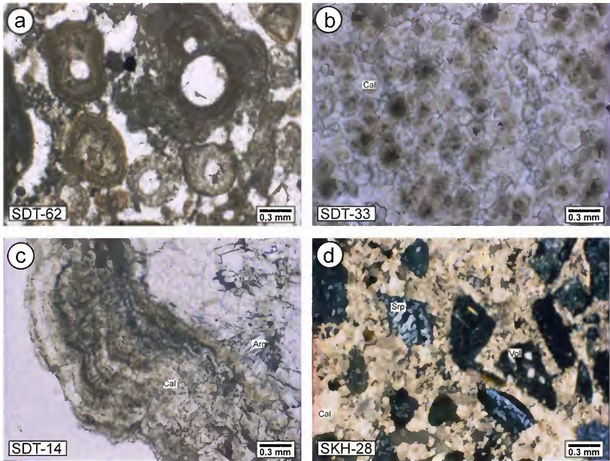
Şekil 4. Karbonat kayaçlarının ve kumtaşının optik mikroskop görünüşleri (tek nikol), a) Oosparitlerde tek ve birleşik oolitler, b) Sparitlerde tanesnel kalsitler, c) Sparitlerde ışınsal aragonitler ve jel dokulu kalsitler, d) Litik grovaplarda serpantin ve volkanik kayaç parçacıkları.
