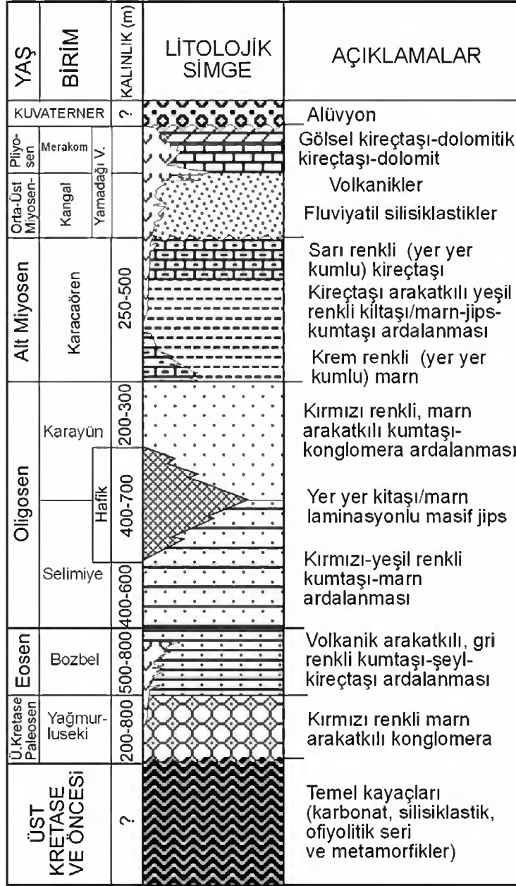
Şekil 3. Sivas ve Kangal havzalarının genelleştirilmiş stratigrafi dikme kesiti.
