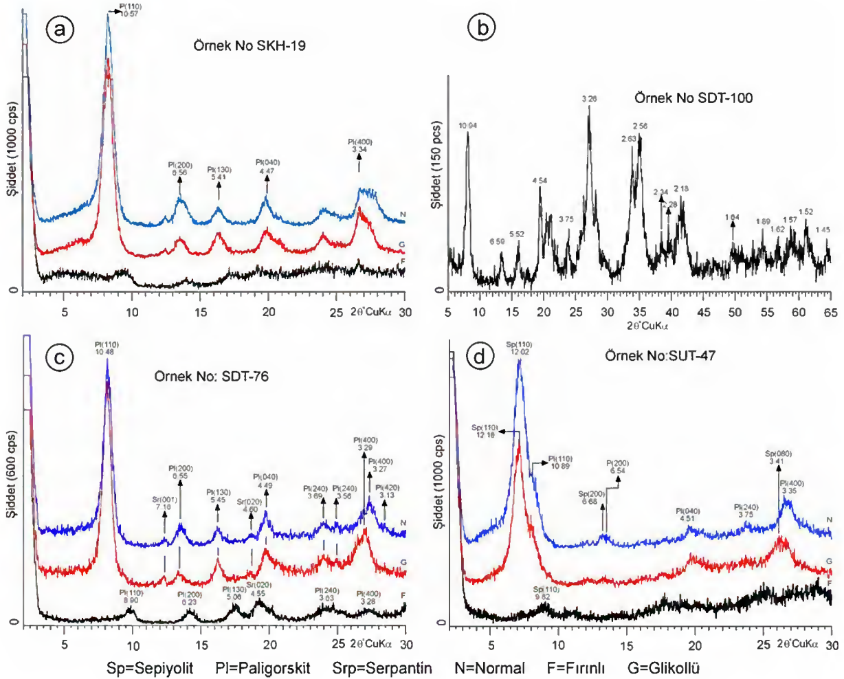
Şekil 7. Kangal Baseni'nde saptanan bazı kil minerallerinin XRD difraktogramları, a) Paligorskit, b) Paligorskit (yönlenebilir), c) Paligorskit+serpantin, d) Sepiyolit + paligorskit.
