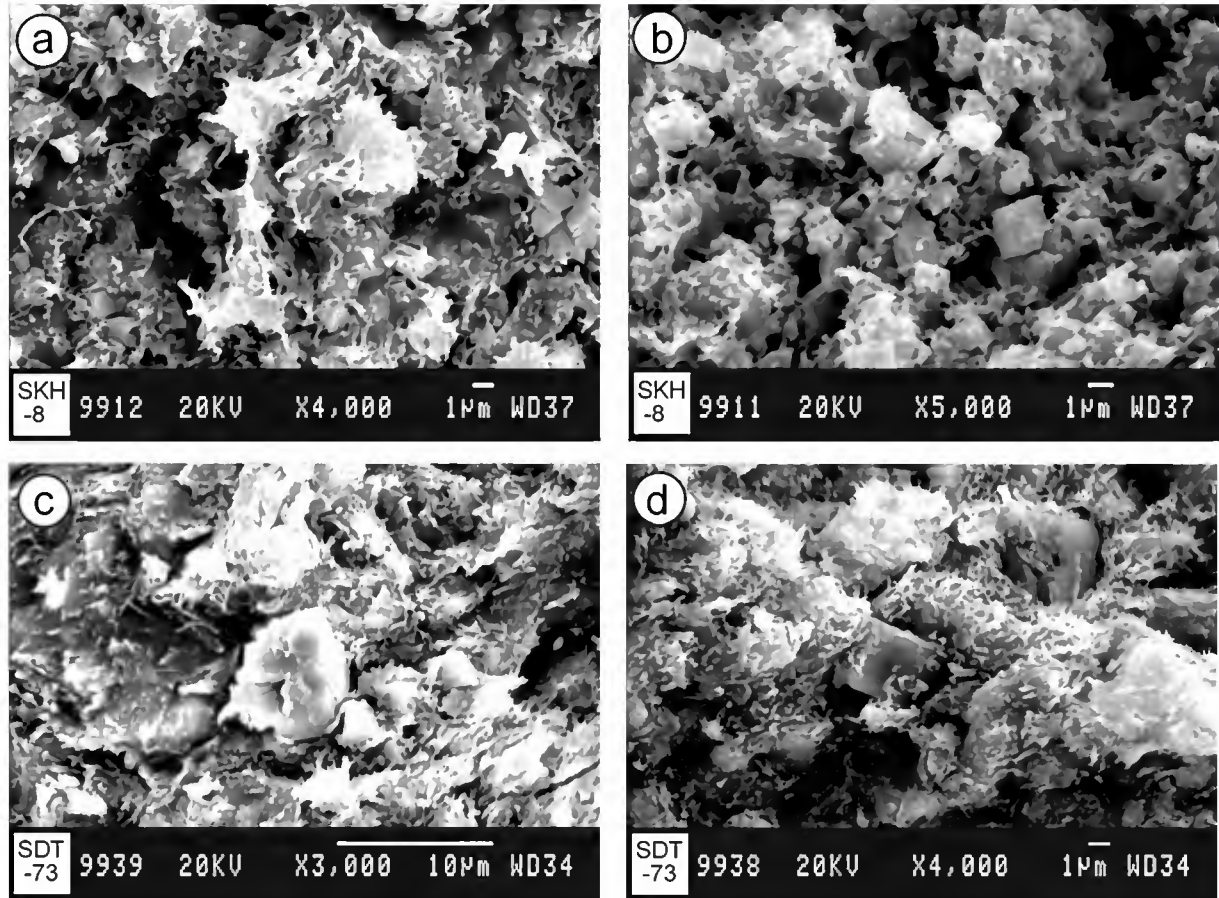
Şekil 5. Dolomitli kireçtaşı (SKH-8) ve killi dolomitlerinin (SDT-73) SEM mikrofotografaları, a) Lifsi sepiyolit-paligorskitler ve karbonat mineralleri, b) Lifsi sepiyolit-paligorskitler ve yer yer çözülmüş karbonat mineralleri (sağ-orta), c) Özşekilli tek ve birleşik dolomitleri çevreleyen lifsi paligorskitler, d) Dolomitlerin üzerinde yer yer büyümüş paligorskitler.
